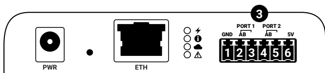
Slika 3: Komunikacijski vtiči RS485 (označeno s številko 3)
